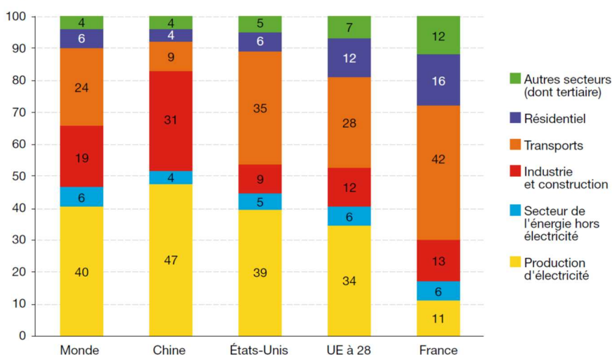
ORIGINE DES ÉMISSIONS DE CO 2 DUES À LA COMBUSTION D'ÉNERGIE EN 2016
